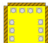
PAN05 Pour 10 bouteilles 2400 x 1760 x 880 mm Poids : 550 kg
