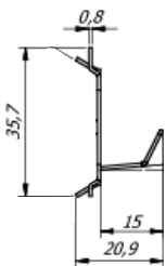
Modèles 70, 100 et 150
