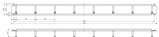
Modèles 160, 224 et 272
