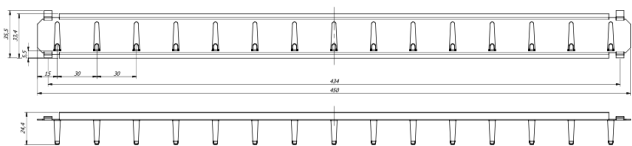
Modèles 300, 420 et 510
