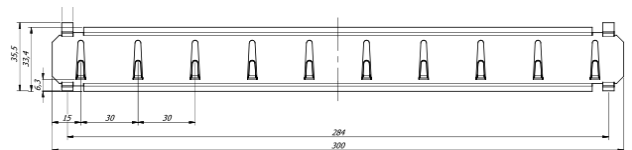
Modèles 70, 100 et 150
