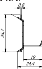
Modèles 160, 224 et 272
