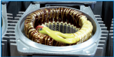
Moteurs à faible vitesse de rotation (1400 trs/min)
