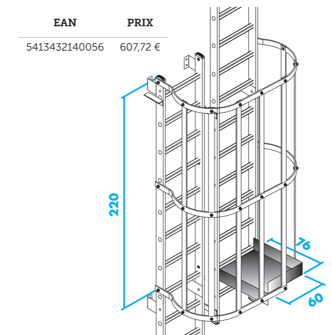
Palier de repos en tôle larmée « brute »
