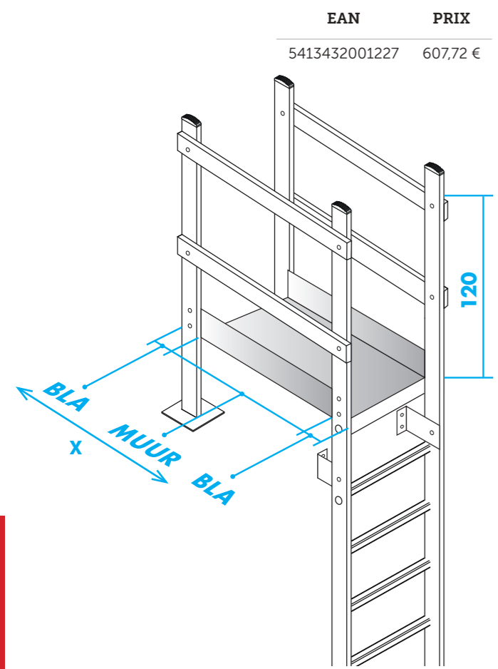
Plateforme de franchissement en tôle larmée « brute » X = 2 X BLA + ÉPAISSEUR DE MUR
