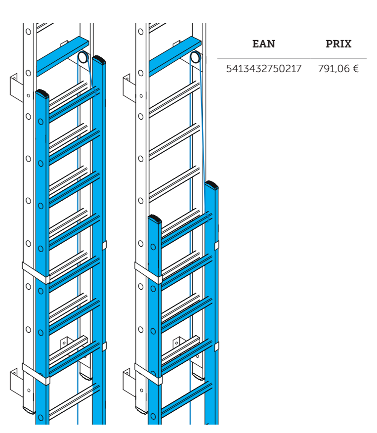
Un chevauchement d'au moins 150 cm est requis.
